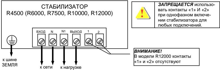
Рисунок 6.1 Схема подключения стабилизатора
